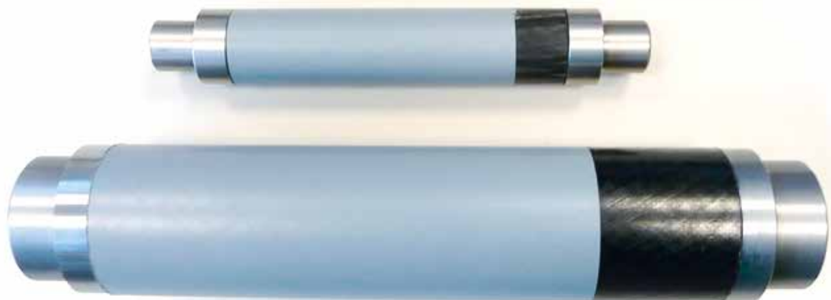
„CFK-Wellen mit lokal applizierter PTFE-Beschichtung (grau)“
